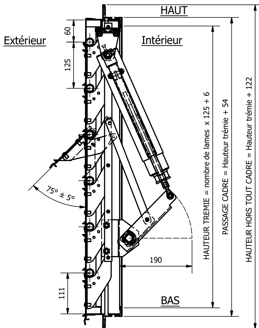
Coupe A-A
